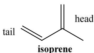
Isoprene
