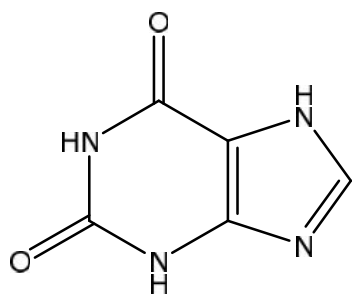
xanthine
