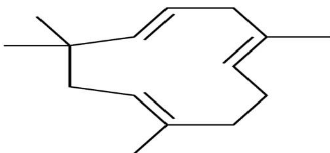
humulene
