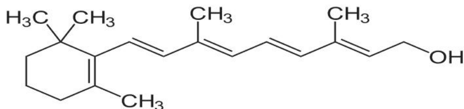
Retinol
