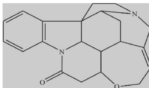
strychnine
