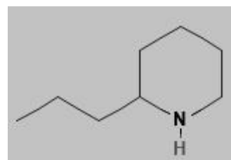
Coniine
