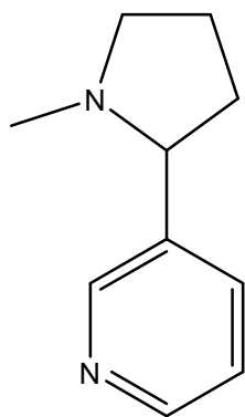
nicotine
